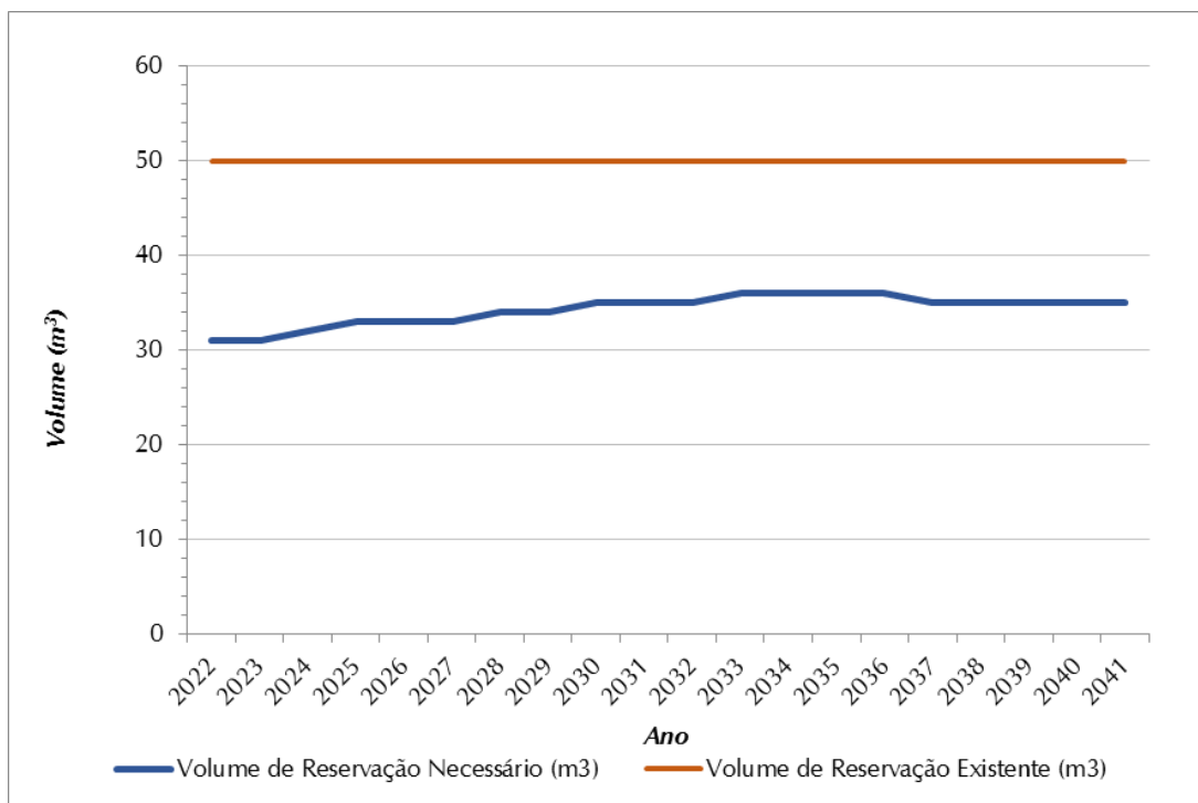
Figura 8.6 - Volume de Reservação Necessário (m³) x Volume de Reservação Atual (m³) - SAA Santa Izabel do Marinheiro
