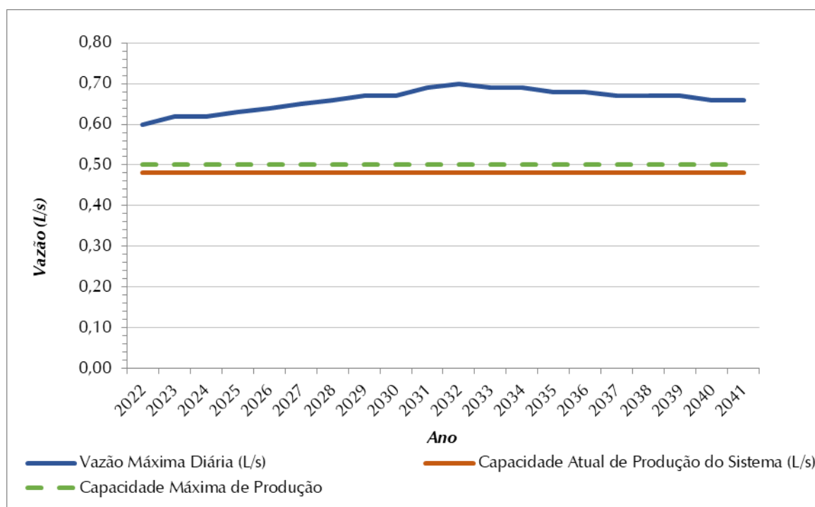
Figura 8.3 – Demandas Máximas Diárias (L/s) X Vazão Captada (L/s) – SAA Dulcelina
