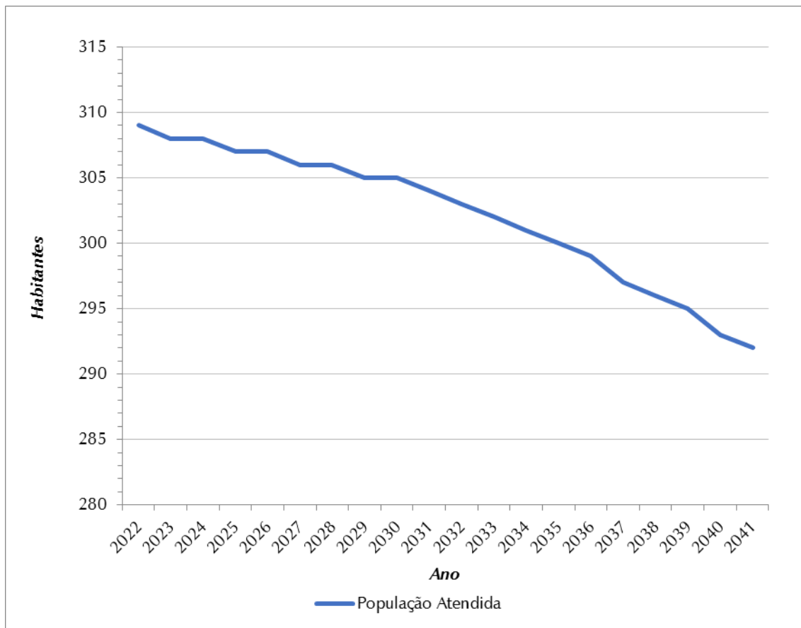
Figura 7.6 - Evolução da População Atendida (hab.) – SES Santa Isabel do Marinheiro
