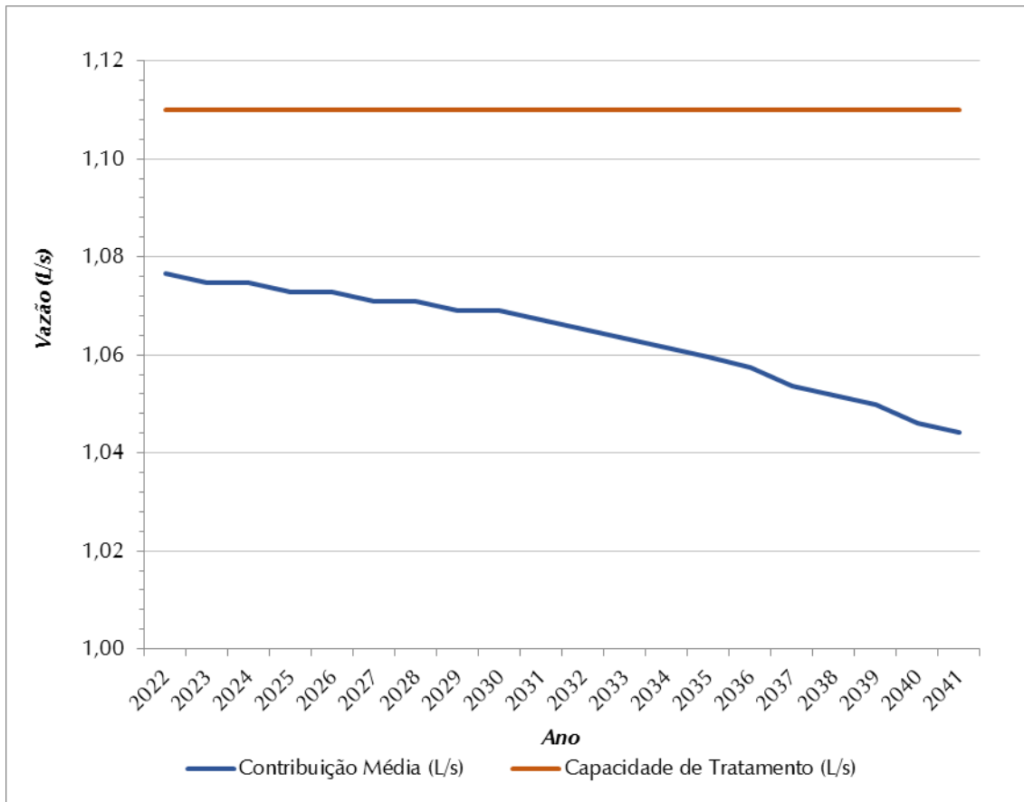
Figura 8.9 – Contribuição Média Total (L/s) x Capacidade de Tratamento de Esgoto (L/s) – SES Santa Izabel do Marinheiro
