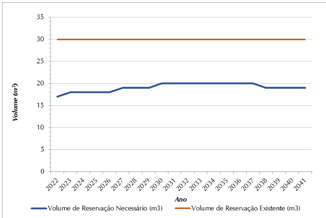
Figura 8.4 - Volume de Reservação Necessário (m³) x Volume de Reservação Atual (m³) - SAA Dulcelina
