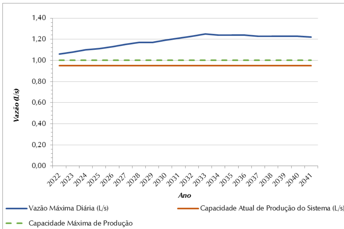
Figura 8.5 – Demandas Máximas Diárias (L/s) X Vazão Captada (L/s) – SAA Santa Izabel do Marinheiro
