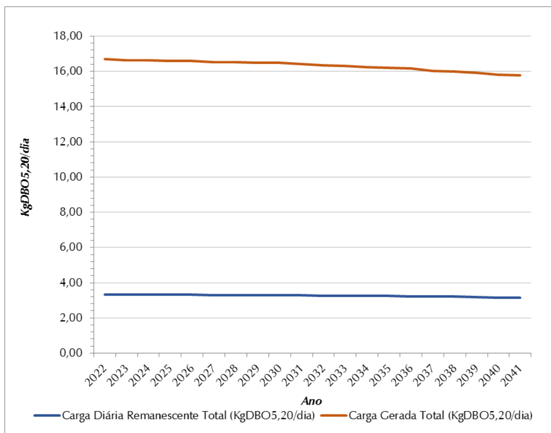
Figura 8.10 - Evolução de Cargas Orgânicas (Kg DBO 5 /Dia) – SES Santa Izabel do Marinheiro
