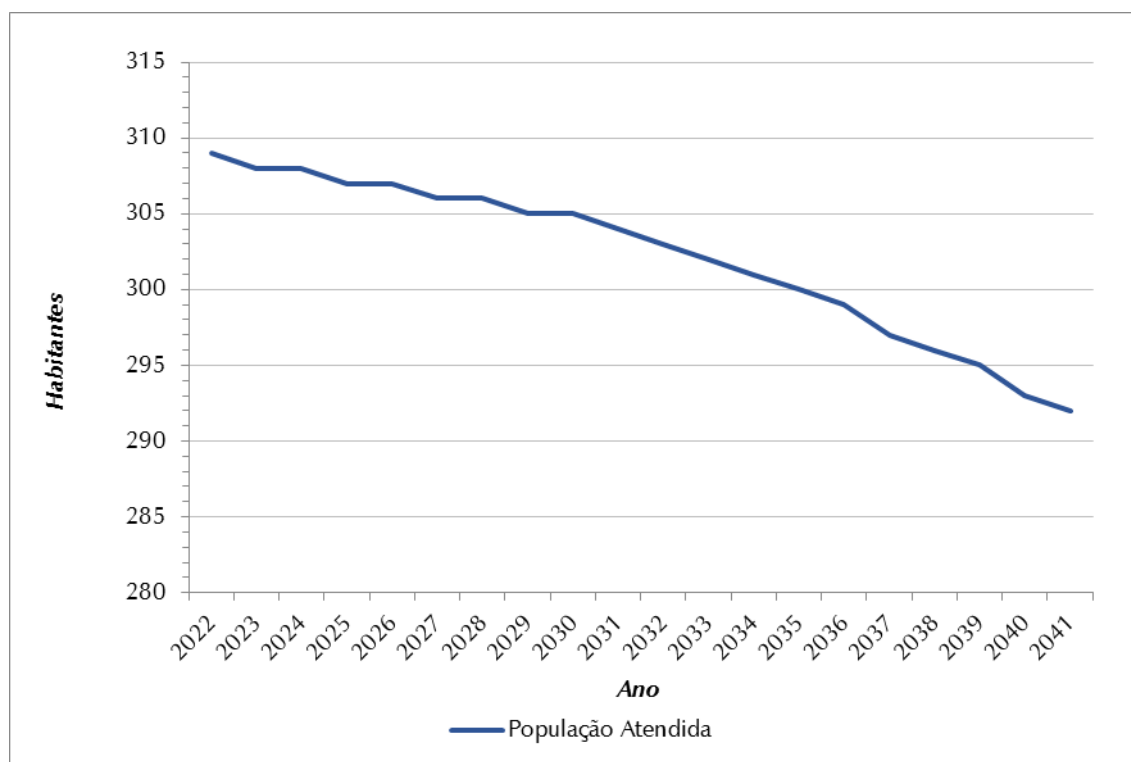
Figura 7.4 – Evolução da População Atendida (hab.) – SAA Santa Izabel
