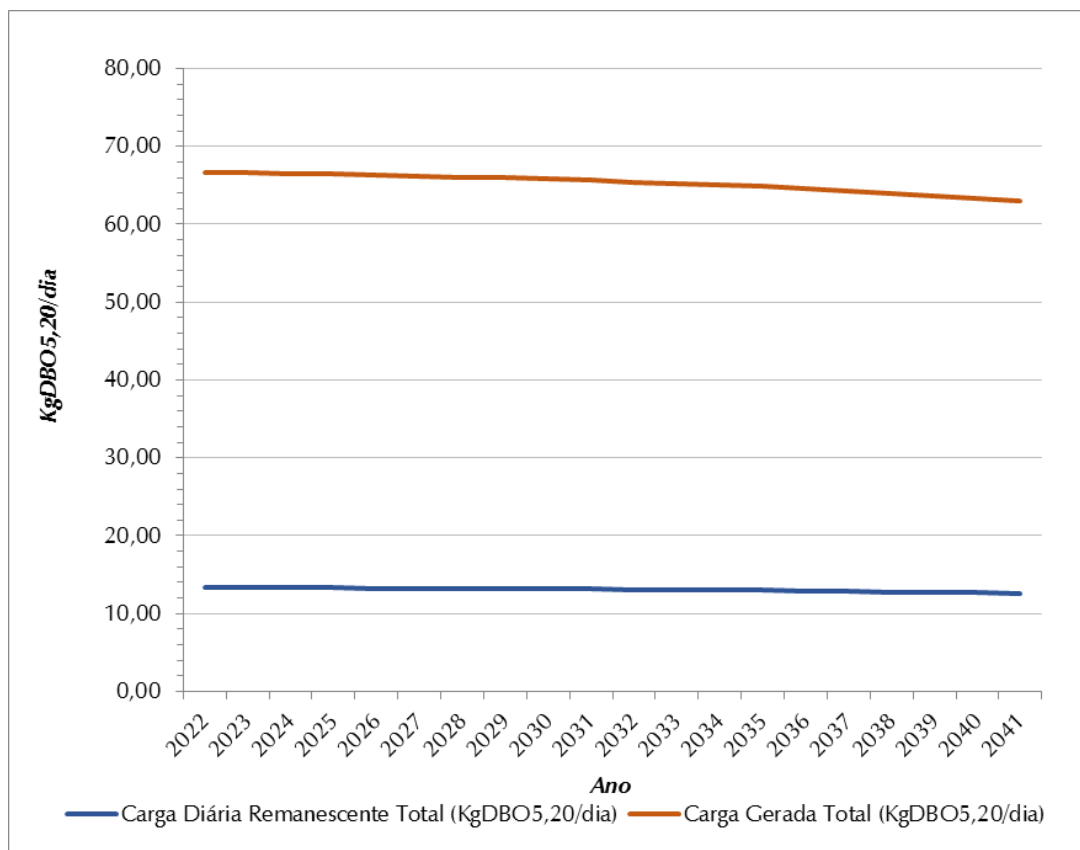
Figura 8.8 - Evolução de Cargas Orgânicas (Kg DBO 5,20 /Dia) – SES Sede
